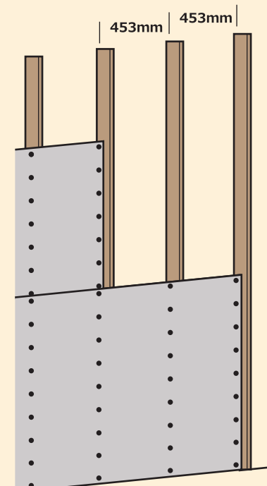
図1：下地の施工
